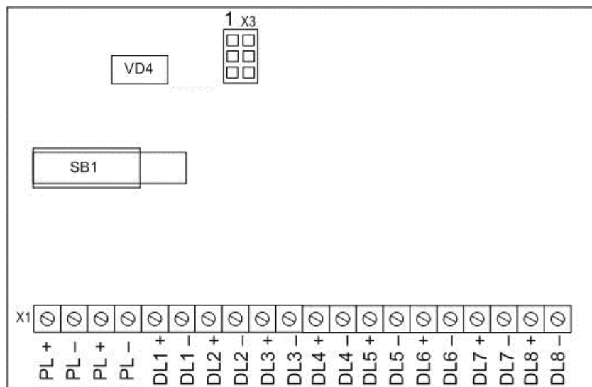
Рисунок 1 – Расположение элементов платы расширителя Elsys-AC-AE8
